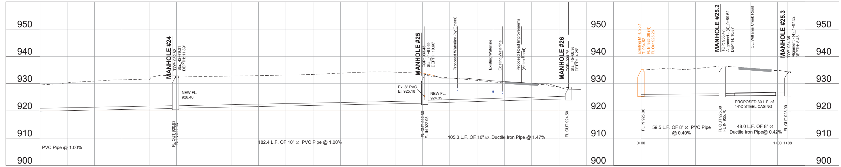
PROFILE SCALE: HORZ. 1"=10' VERT. 1"=5'
